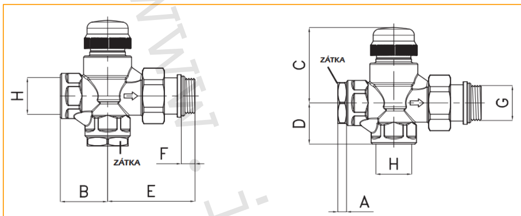
Provedení přímé – zátko dole
