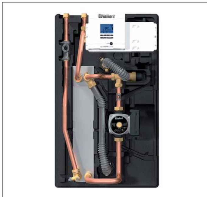
Jednotka k ohřevu teplé vody aquaFLOW exclusive VPM W
