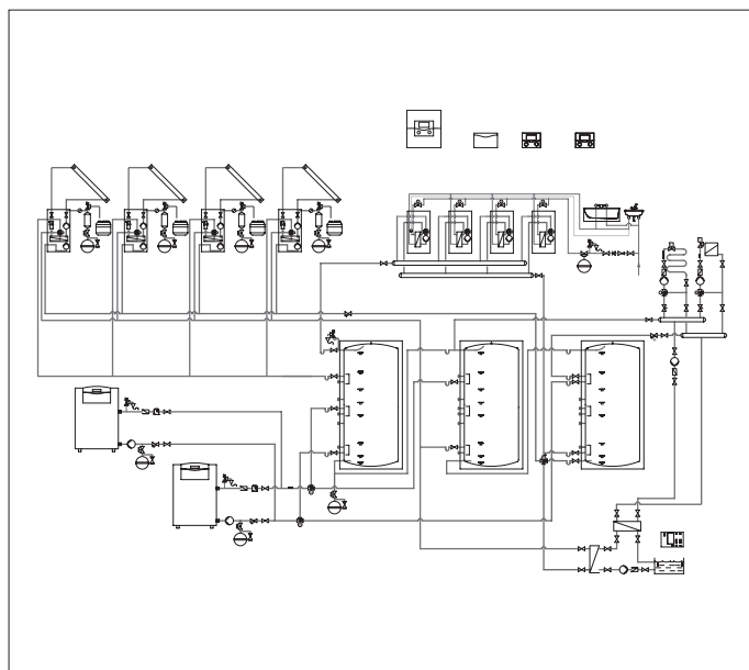
Náhled systému 4
