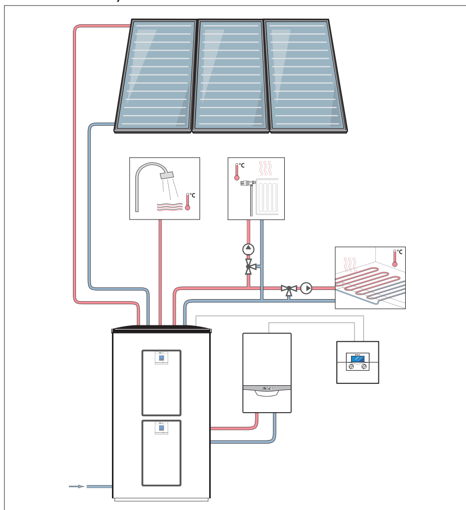
Akumulační systém allSTOR
