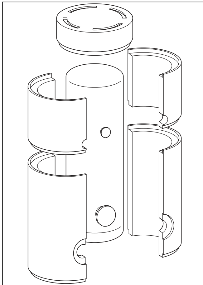
Obr. 5.11 Odobratie izolácie
