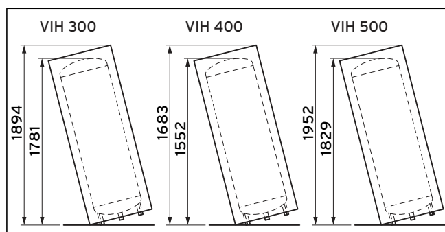
5.1 ábra VIH R, VIH S és VIH RW döntési méretek
