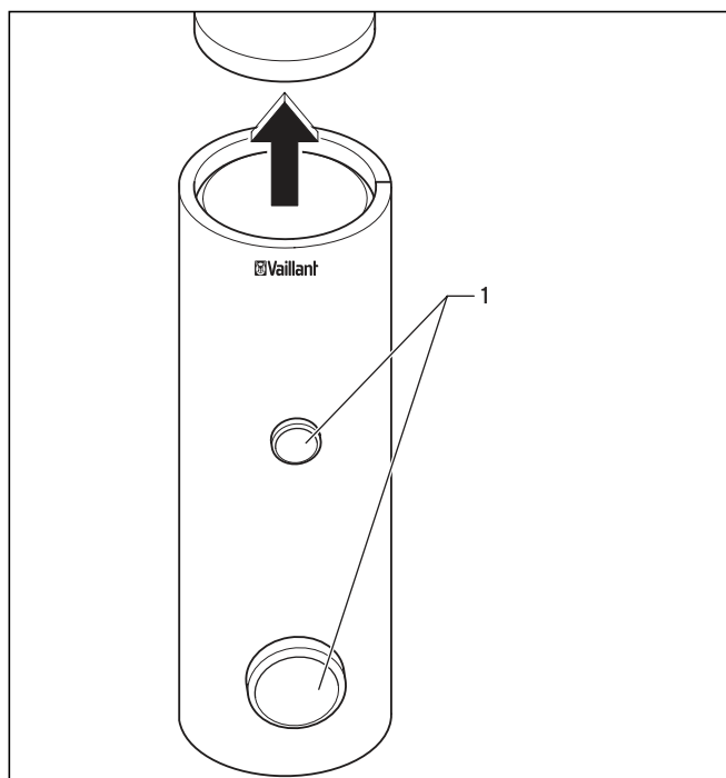
Rys. 5.7 Zdjąć pokrywę i osłony
