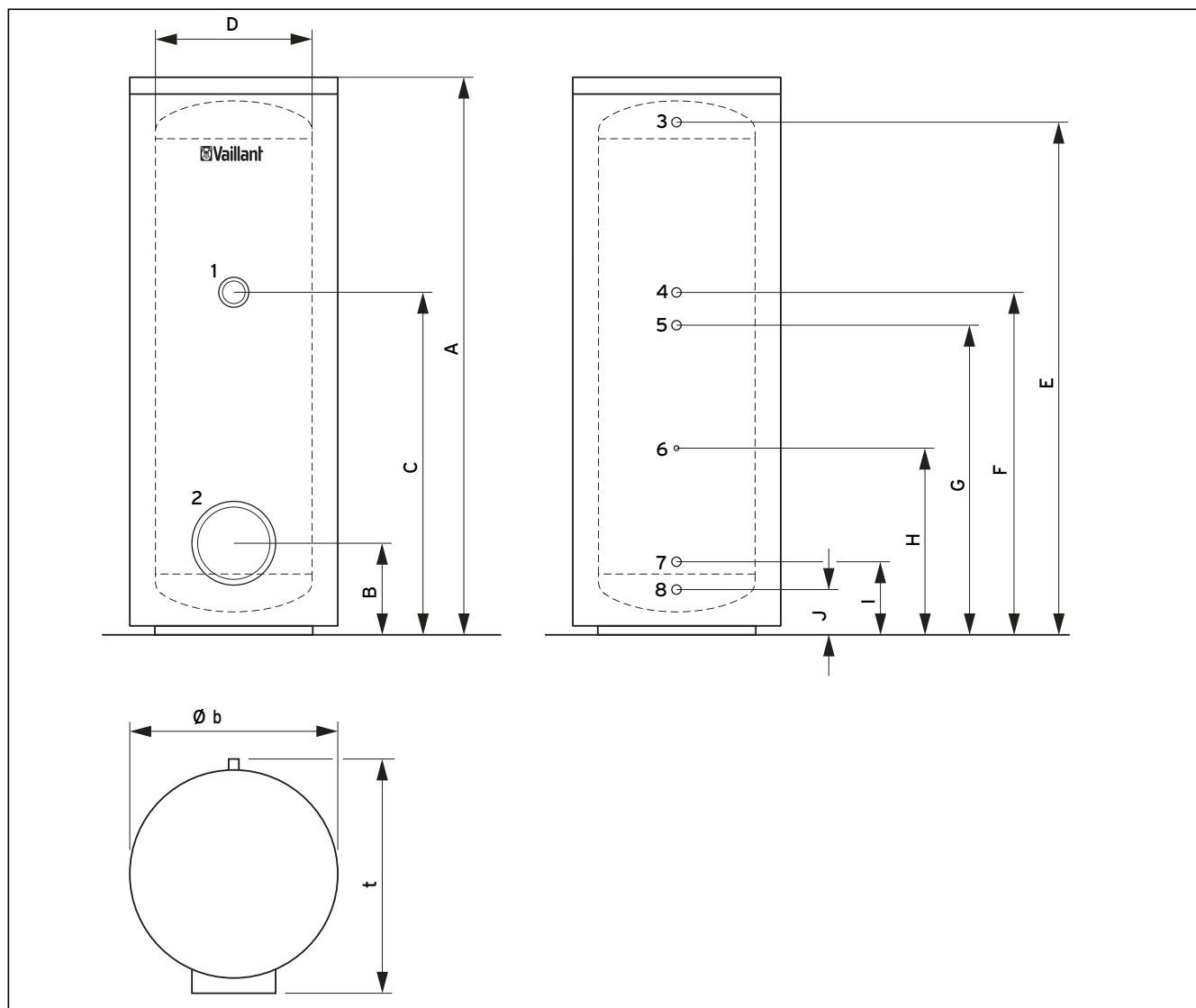
5.3 ábra VIH R készülék- és csatlakozóméretetek
