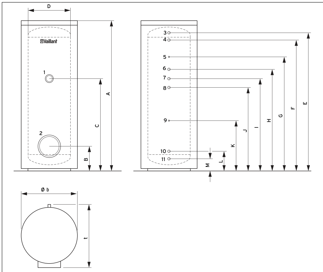
Rys. 5.2 Wymiary gabarytowe i przyłączone zasobnika VIH S
