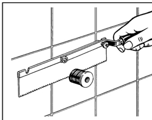
Verkröppte Handsäge
