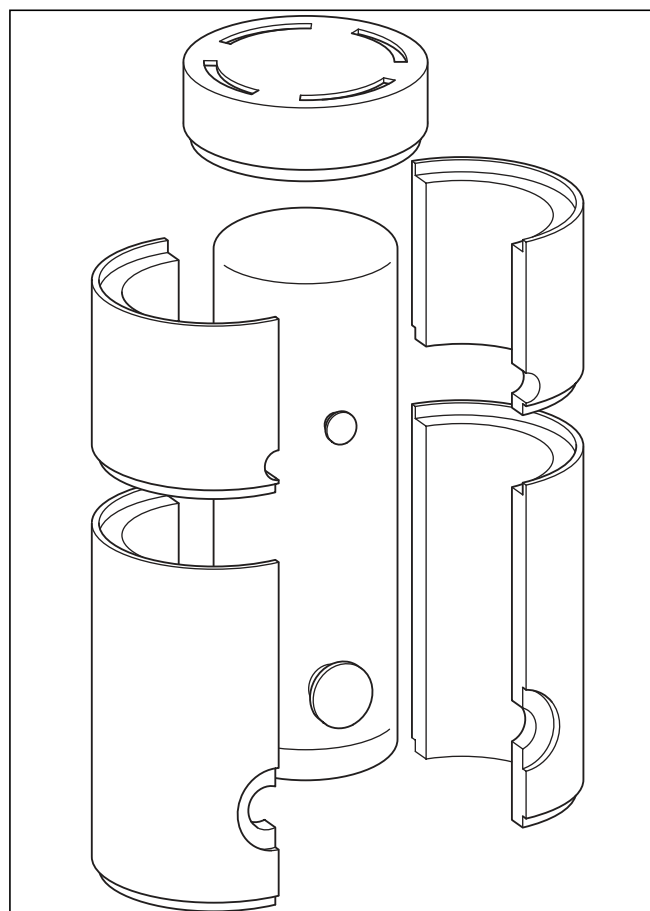
Obr. 5.9 Demontáž izolace
