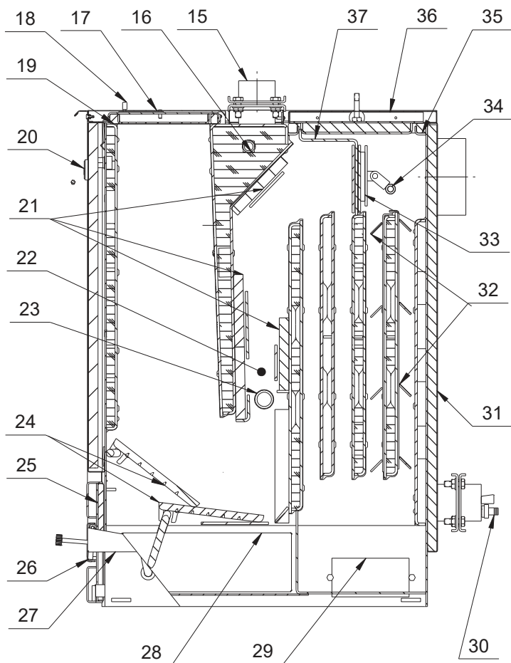
Obr. 4 Schéma kotle SL27E
