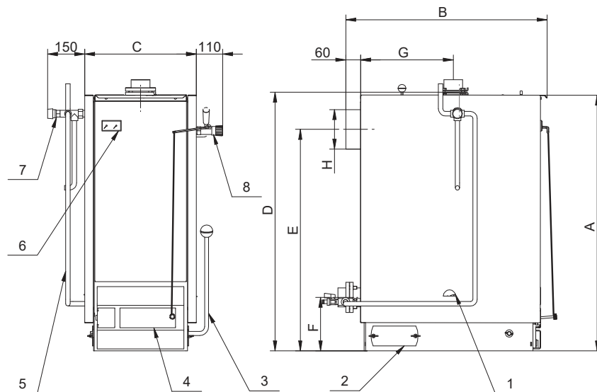
Obr. 1 Hlavní rozměry kotle SL14E, SL20E, SL27E
