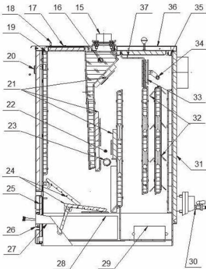
Obr. 3 Schéma kotle SL20E
