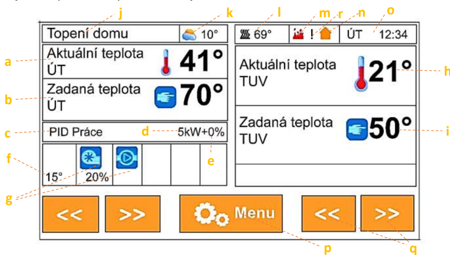
Hlavní panel řídicí jednotky v9 MINI
