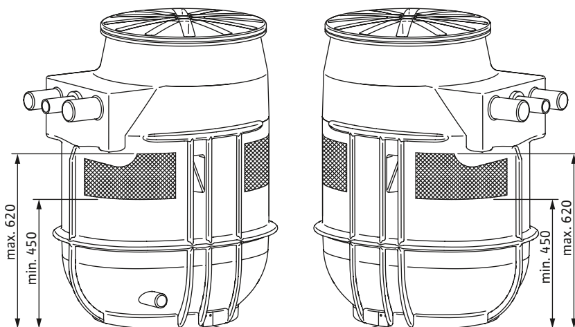
Fig. 9: Přítokové plochy
