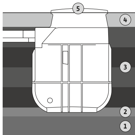
Fig. 23: Zасыпání příkopu
