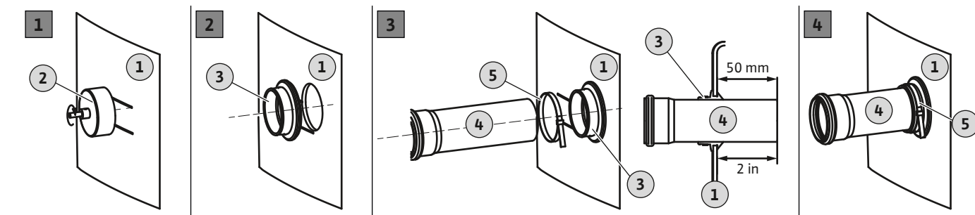
Fig. 10: Připojení přítoku
