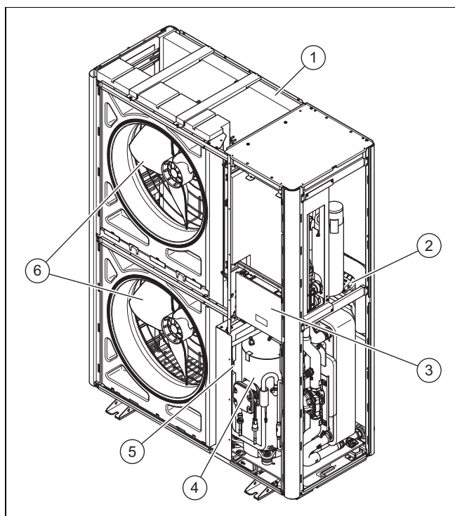
1 Parowacz 2 Płytki elektroniczne INSTALLER BOARD 3 Płytki elektroniczne HMU 4 Podzespół sprężarki 5 Zespół konstrukcyjny INVERTER 6 Wentylator
