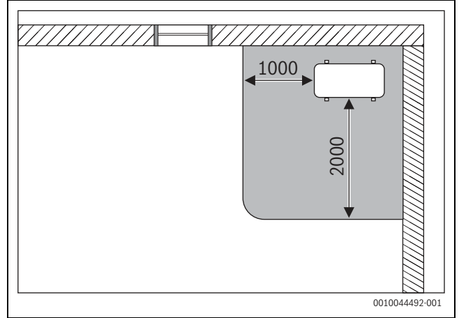
Res. 72 Koruma bölgesi, bir köşeye yaslanmış ayaklı dış ünite - ölçüler (mm)
