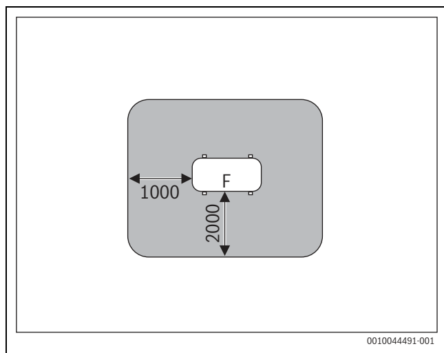
Σχ. 14 Προστατευμένη περιοχή κατά την τοποθέτηση στο δάπεδο στο οικοπέδο ή την οροφή - διάσταση σε mm
