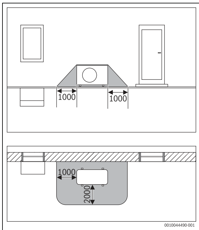
fig. 64 Zona e mbrojtjes, njësi e jashtme me qëndrim në dyshe me një mur - përmasat në mm
