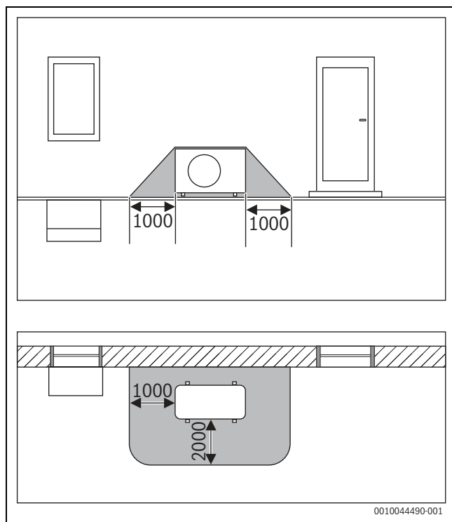
Obr. 58 Ochranná zóna, vonkajšia jednotka postavená na podlahe pri stene – rozmery v mm
