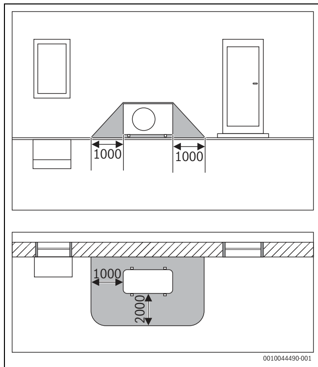
Rys. 49 Strefa ochronna, jednostka zewnętrzna posadowiona na gruncie przy ścianie – wymiary w mm
