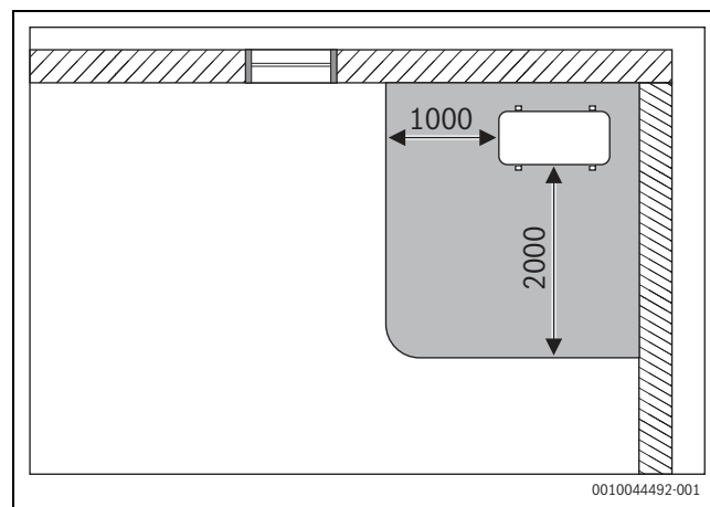
Σχ. 15 Προστατευμένη περιοχή, εξωτερική μονάδα τοποθετημένη στο δάπεδο σε γωνία - απόσταση σε mm
