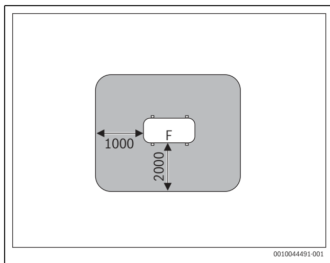
Joon. 23 Ohupiirkond paigaldusel kinnistul maapinnale või katusele – mõõdud mm-tes
