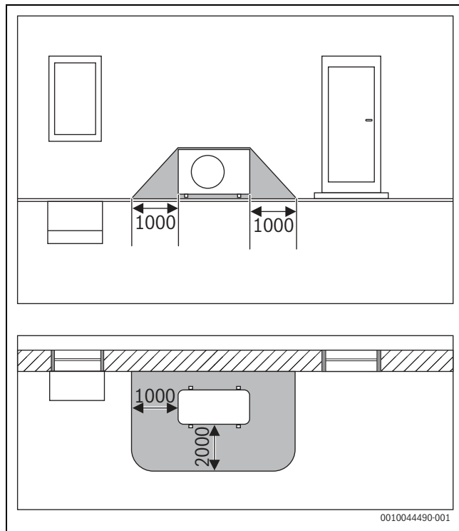
Joon. 22 Ohupiirkond, seinä ääres põrandal seisva välisseadme – mõõdud mm-tes
