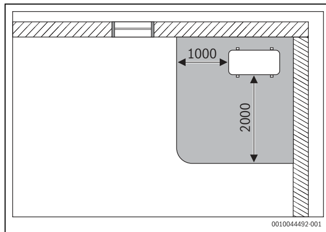
Rys. 51 Strefa ochronna, jednostka zewnętrzna posadowiona na gruncie w narożniku – wymiary w mm
