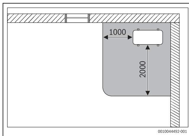
Сл. 45 Заштитено подрачје, подна надворешна единица со димензии на агол во mm
