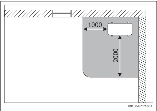
Fig. 54 Área de proteção, unidade exterior de chão num canto - Dimensões em mm
