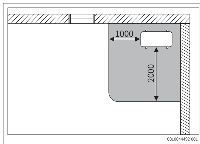
Obr. 60 Ochranná zóna, vonkajšia jednotka postavená na podlahe v rohu – rozmery v mm
