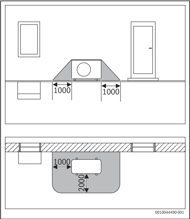
Fig. 52 Área de proteção, unidade exterior de chão numa parede - Dimensões em mm
