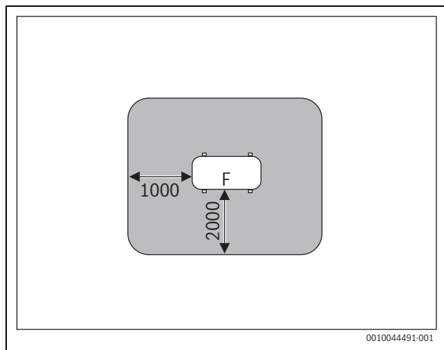
Fig. 26 Volume de protection pour la mise en place au sol sur le terrain ou le toit - dimensions en mm
