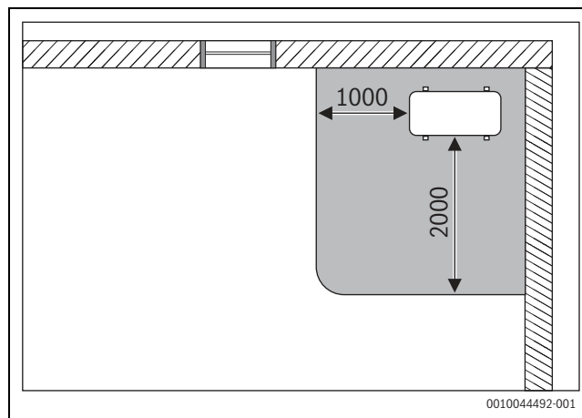
Sl. 30 Zaštitno područje, samostojeća vanjska jedinica u kutu - dimenzije u mm
