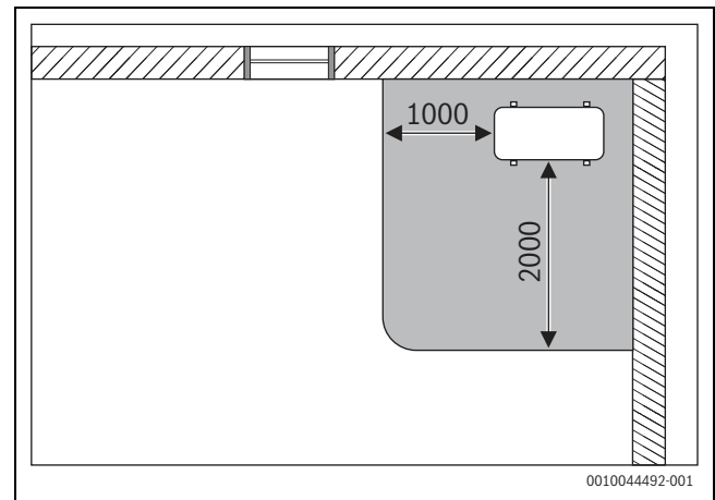
Joon. 24 Ohupiirkond, nurgas põrandal seisva välisseadme – mõõdud mm-tes
