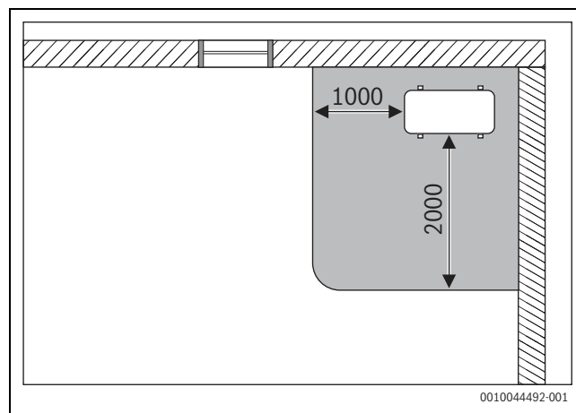
Fig. 36 Zona di sicurezza, unità esterna a basamento installata in un angolo - misure in mm
