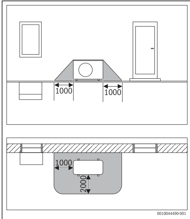
Fig. 7 Sikkerhedsområde, udvendig enhed stående på jorden op ad en væg – mål i mm
