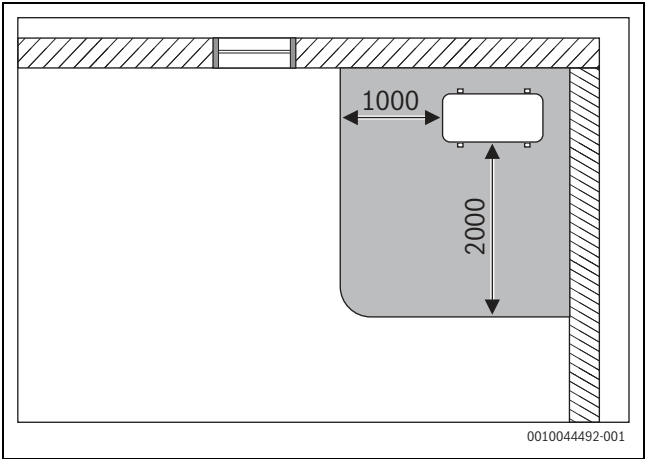
Fig. 21 Sector de protección en unidad exterior situada en el suelo en una esquina - medida en mm
