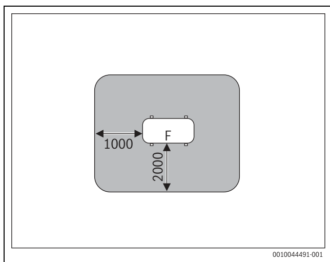
Fig. 35 Zona di sicurezza per installazione a pavimento sul terreno di pertinenza o sul tetto - misure in mm
