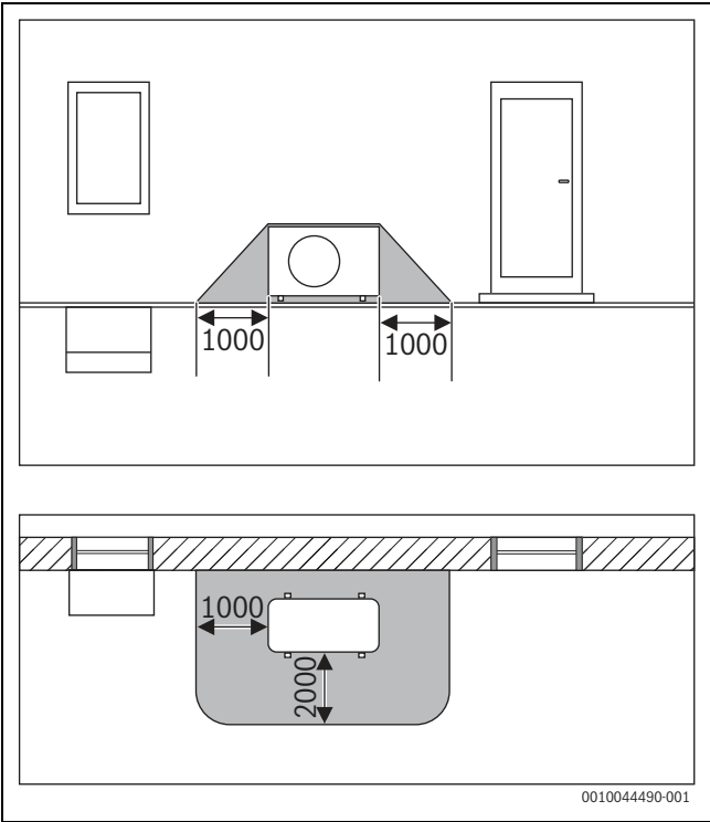
Fig. 19 Sector de protección en unidad exterior situada en el suelo a una pared - medida en mm
