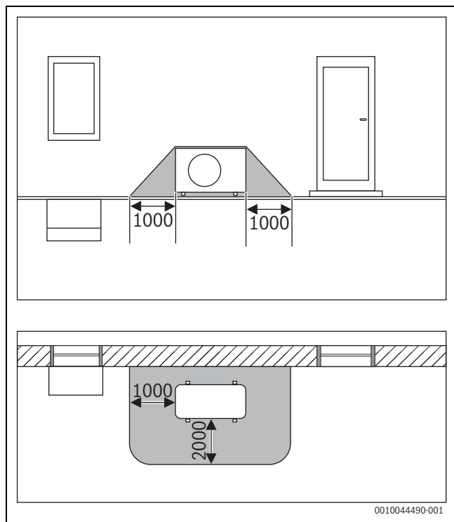
Sl. 28 Zaštitno područje, samostojeća vanjska jedinica na zidu - dimenzije u mm
