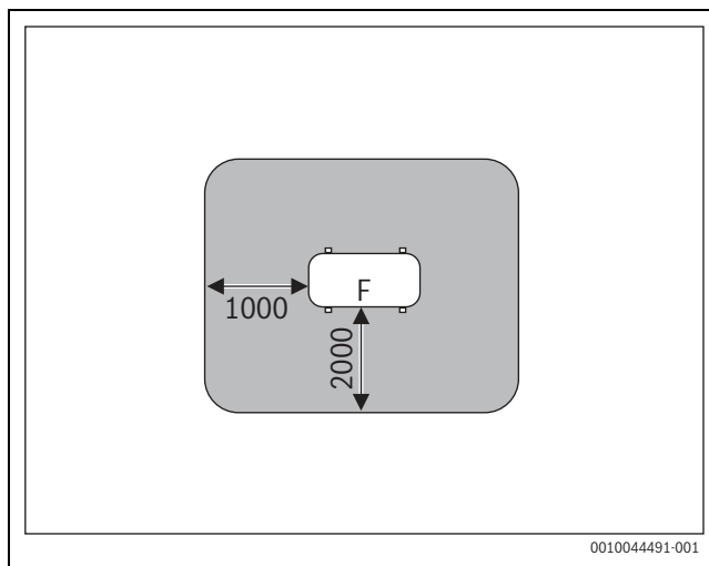
Мал. 74 Захисна зона в разі встановлення на землю на ділянці або даху – розміри в мм
