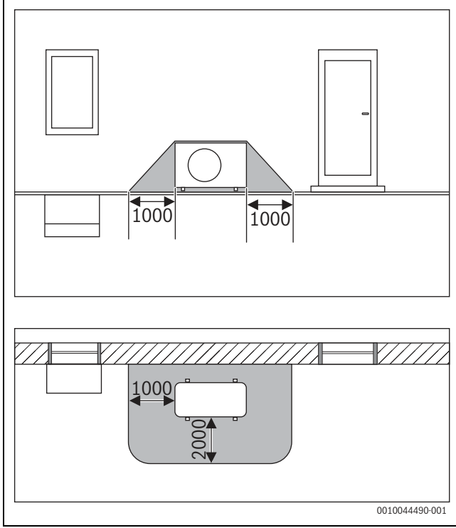
Res. 70 Koruma bölgesi, bir duvara yaslanmış ayaklı dış ünite - ölçüler (mm)
