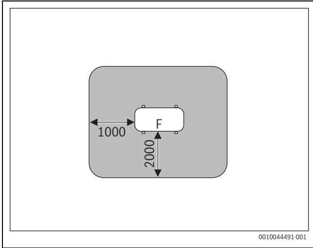
Res. 71 Dış ünitenin arazi veya tavan zemin üzerine yerleştirilmesi durumunda koruma bölgesi - ölçüler (mm)
