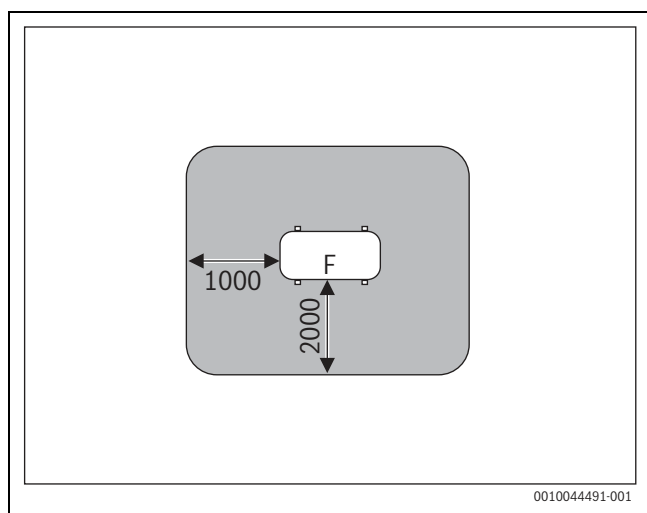
Afb. 47 Veiligheidszone bij opstelling op de vloer op het terrein of dak - maten in mm
