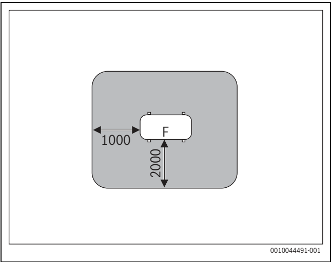
Fig. 53 Área de proteção com instalação no chão na propriedade ou no telhado - Dimensões em mm
