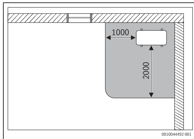
Att. 42 Aizsardzības zona, uz grīdas novietots ārējais bloks stūrī – izmēri mm
