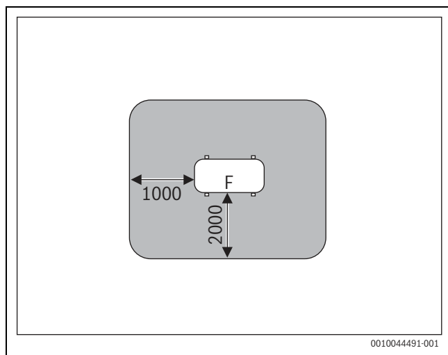
Rys. 50 Strefa ochronna dla urządzenia ustawionego na gruncie na parceli lub na dachu – wymiary w mm
