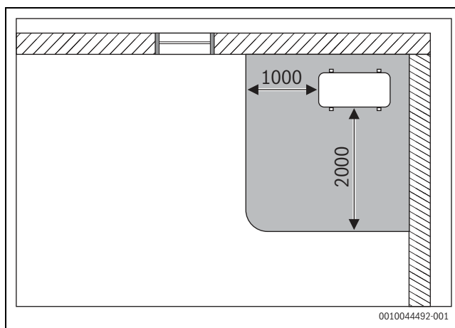
Мал. 75 Захисна зона із зовнішнім підлоговим блоком у куті – розміри в мм
