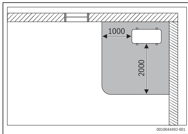
Afb. 48 Veiligheidszone, vloerstaande buitenunit in een hoek - maten in mm
