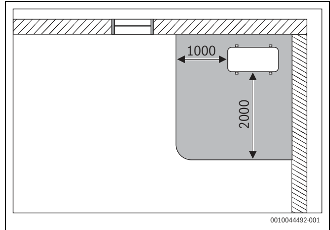
Fig. 9 Sikkerhedsområde, udvendig enhed stående på jorden i et hjørne – mål i mm
