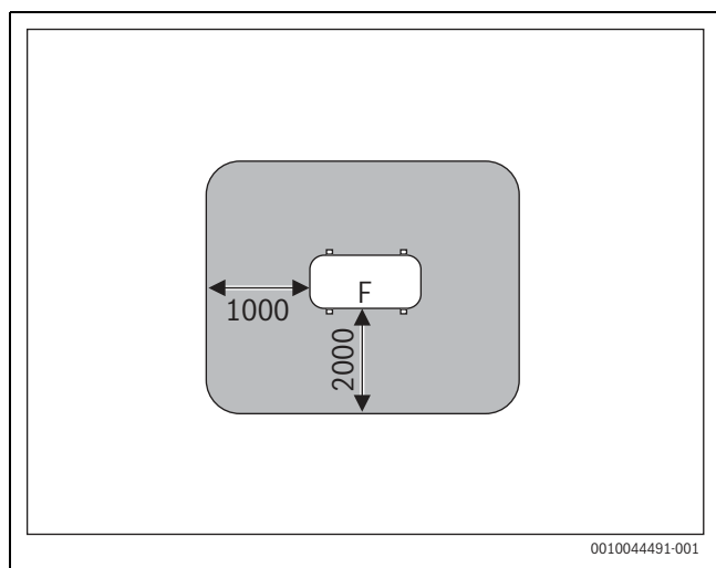
Sl. 29 Zaštitno područje u slučaju postavljanja na pod na zemljištu ili krovu - dimenzije u mm
