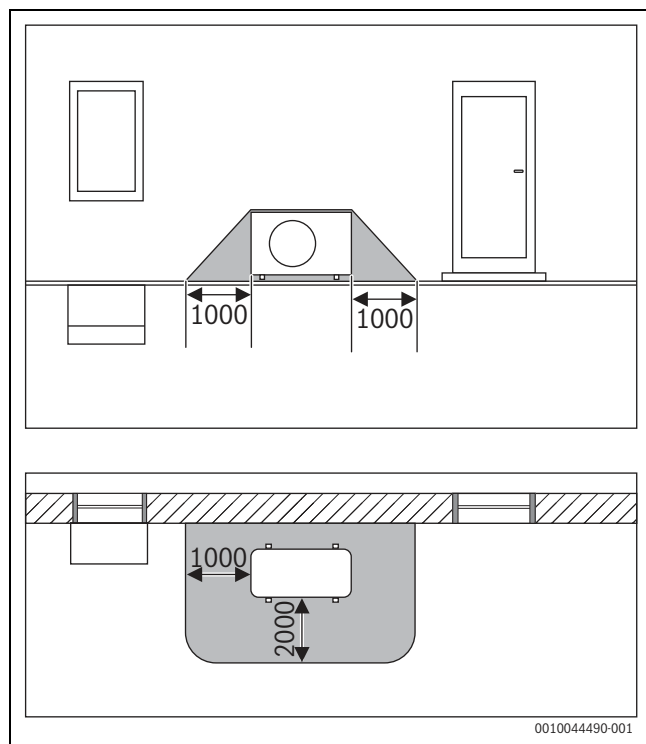
Сл. 43 Заштитено подрачје, подна надворешна единица на сид димензии на сид во mm
