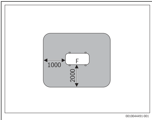
Sl. 62 Varnostno območje pri postavitvi na tla na zemljišču ali strehi – mere v mm
