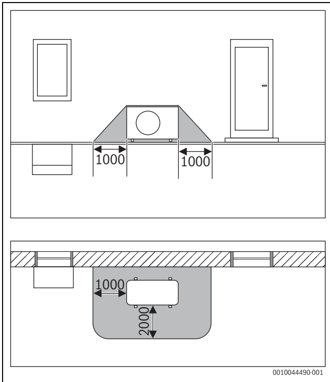
Sl. 61 Varnostno območje, talna zunanja enota na steni – mere v mm
