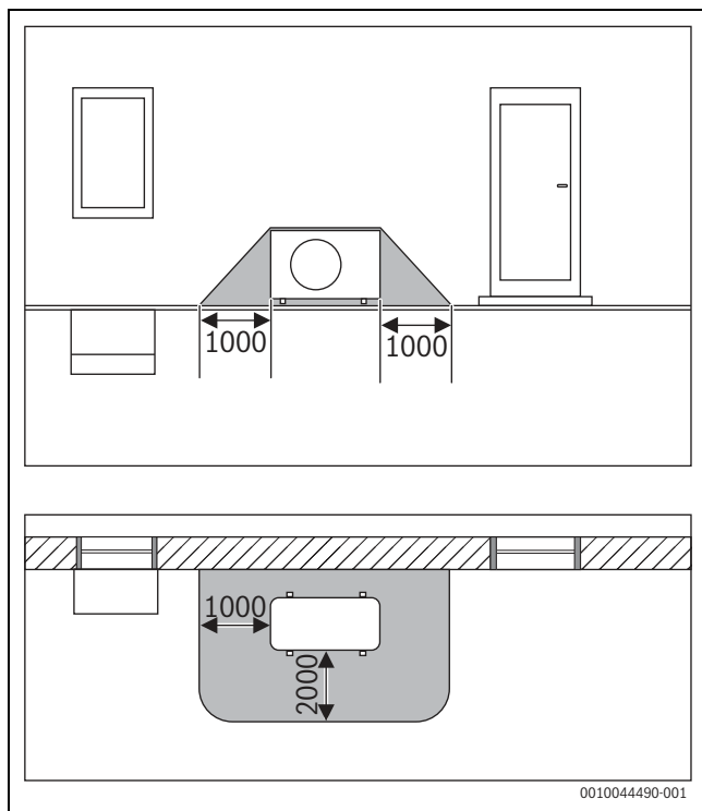
Bild 10 Schutzbereich, bodenstehende Außeneinheit an einer Wand (Maße in mm)
