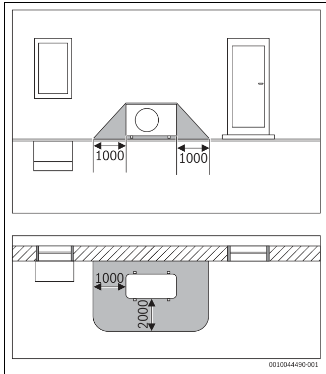
Fig. 25 Volume de protection, unité extérieure au sol contre un mur - dimensions en mm
