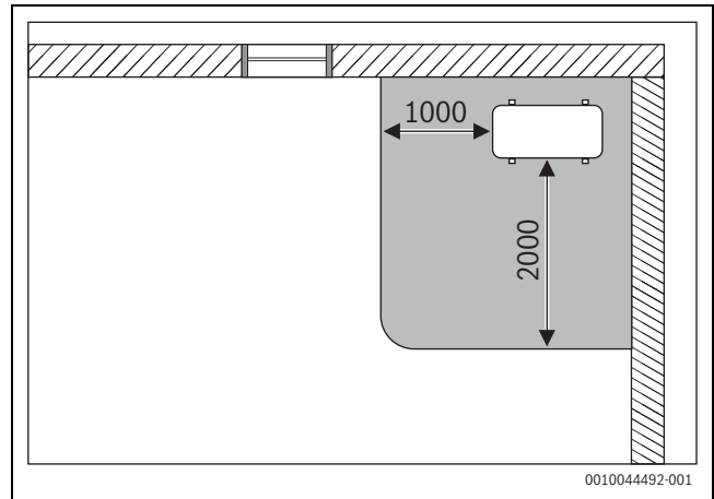
sl. 69 Zona zaštite, stojeća spoljna jedinica u uglu - dimenzije u mm
