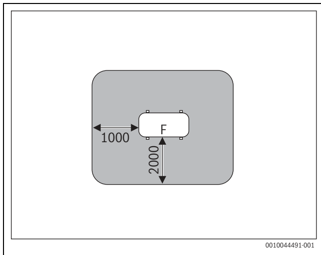
Fig. 8 Sikkerhedsområde ved opstilling på jorden på grundstykket eller på tag – mål i mm
