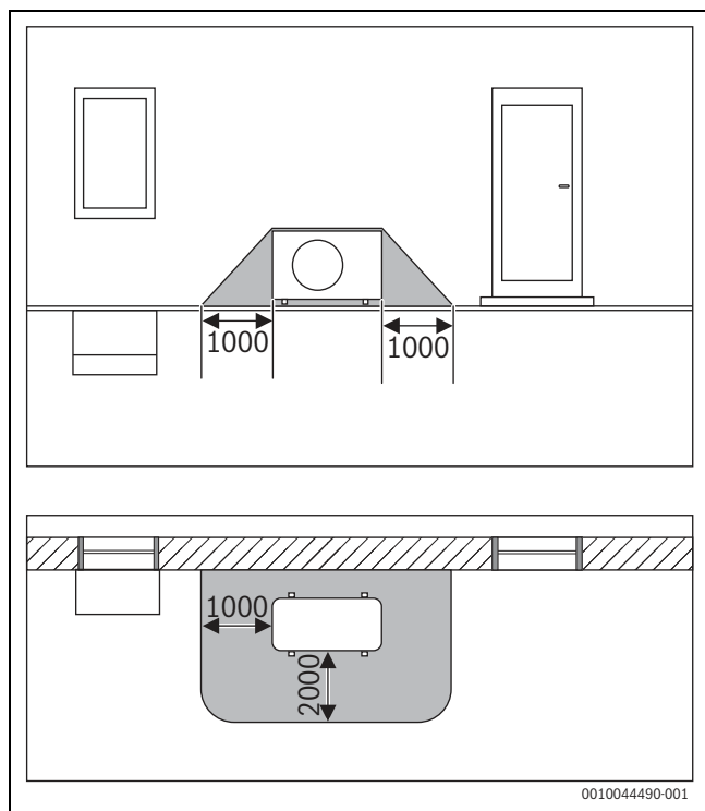
Afb. 46 Veiligheidszone, vloerstaande buitenunit op een wand - maten in mm
