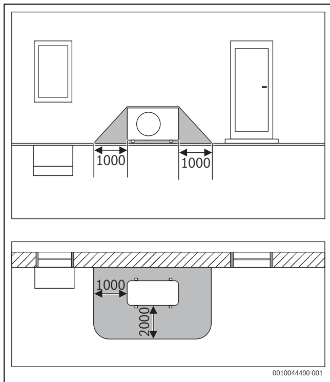
Fig. 34 Zona di sicurezza, unità esterna a basamento installata a ridosso di una parete - misure in mm
