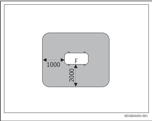
Fig. 20 Sector de protección en caso de posición sobre el suelo en el inmueble o tejado - medidas en mm
