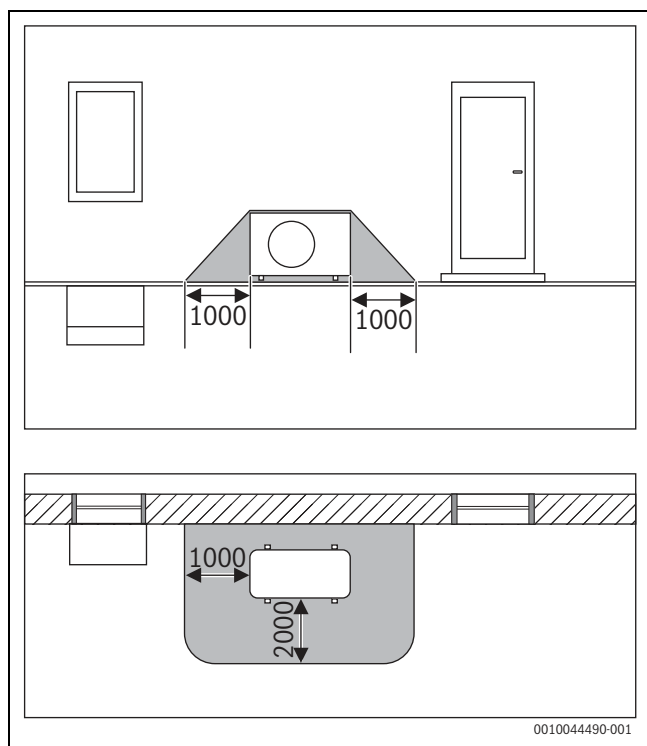
Мал. 73 Захисна зона із зовнішнім підлоговим блоком на стіні – розміри в мм
