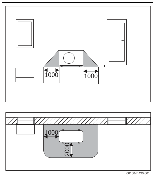
Σχ. 13 Προστατευμένη περιοχή, εξωτερική μονάδα τοποθετημένη στο δάπεδο σε γωνία - απόσταση σε mm
