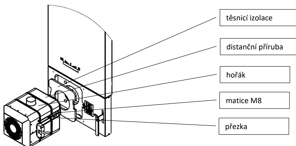
Instalace peletového hořáku do dvířek kotle
