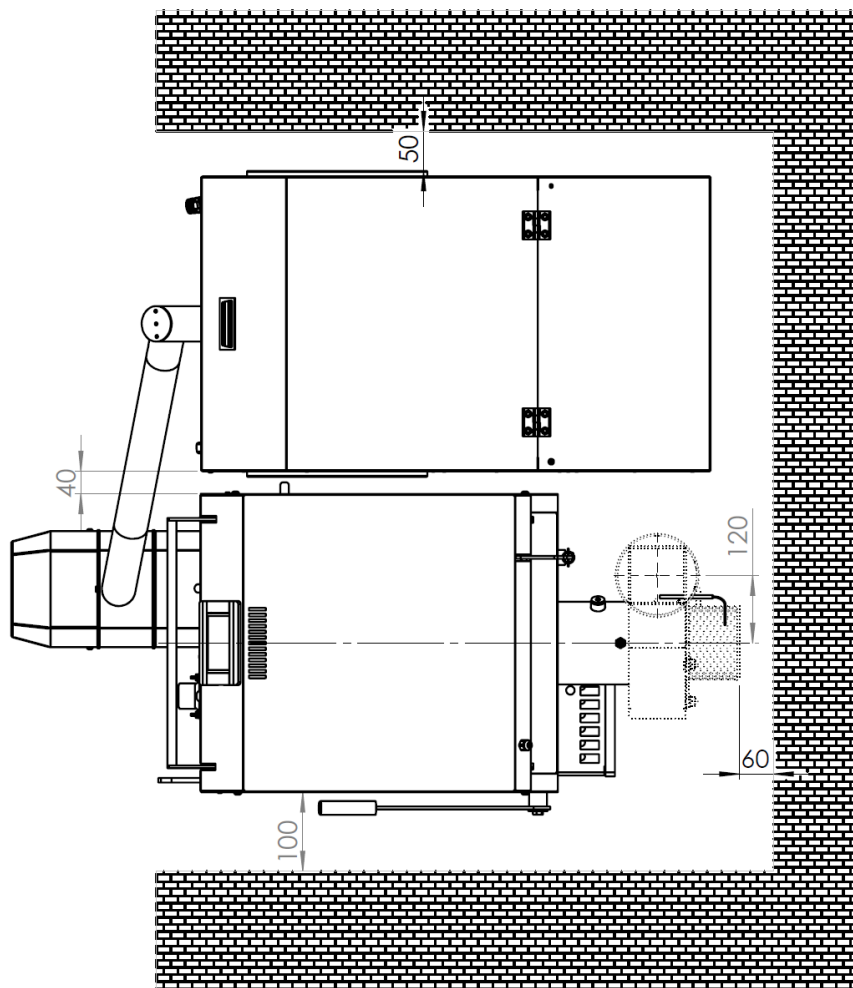
Minimální rozměry při umístění kotle
