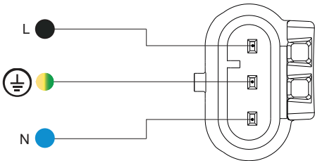
Síťová zástrčka
