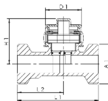
Fig. 138 6 G, DN 10 - DN 50
