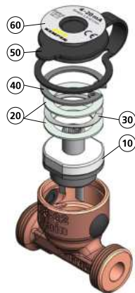
DN 15 - 32 DN 40 - 50 (ohne Abbildung)
